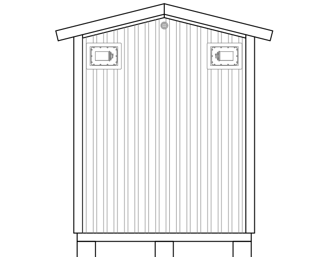
Julkisivu C.-B.
