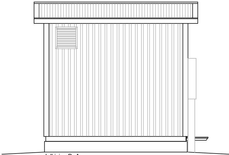
Julkisivu B.-A.
