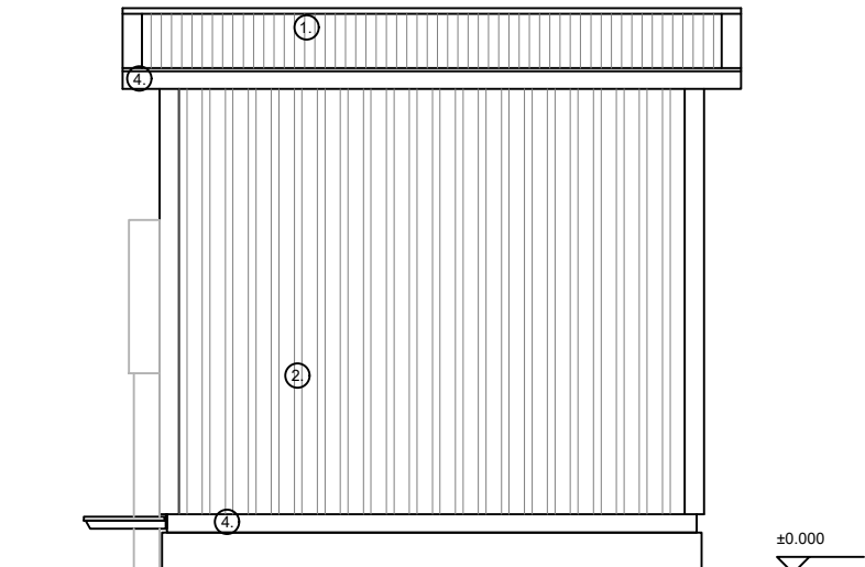
Julkisivu D.-C.
