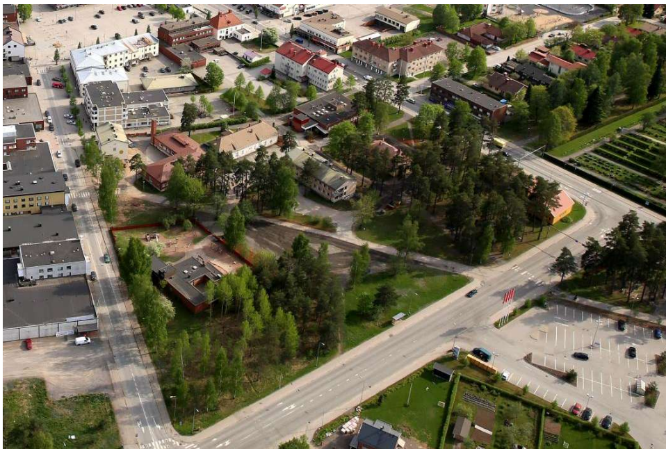
Kuva 20 Viistoilmakuva suunnittelualueelta.
