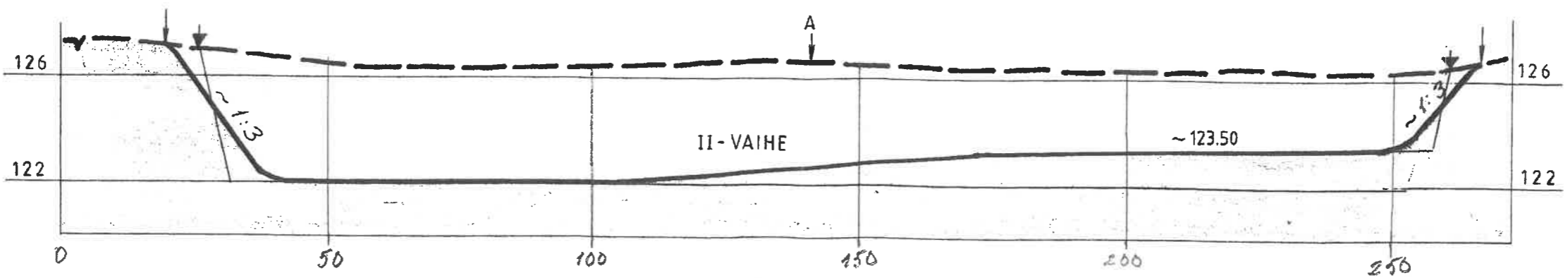
Leikkaus C - C
